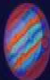
JUPITER
