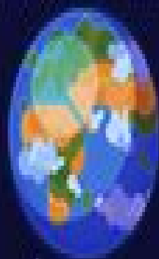
TRES-4B
