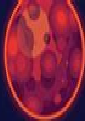
WOLF 359
